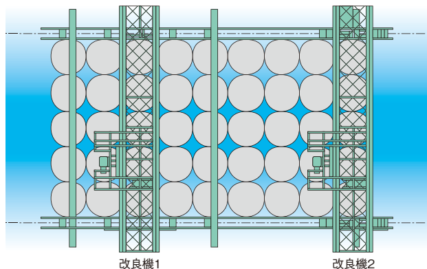
▲ 施工平面図例
